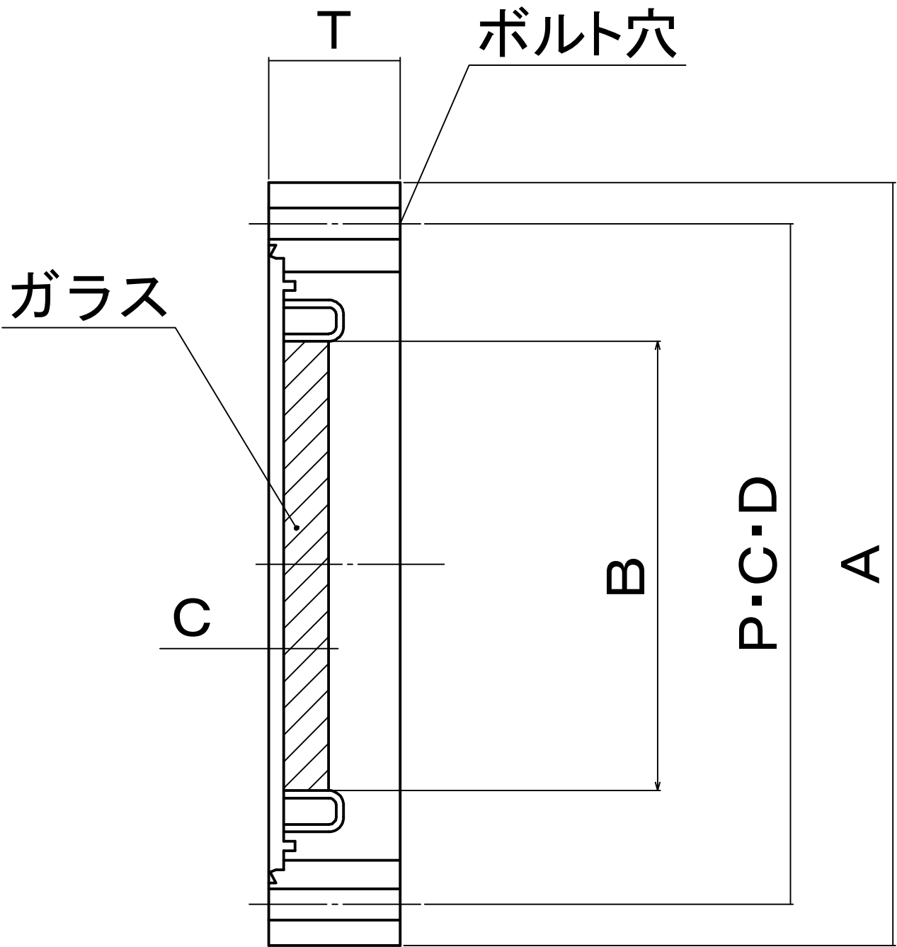
CFガラスビューポート
