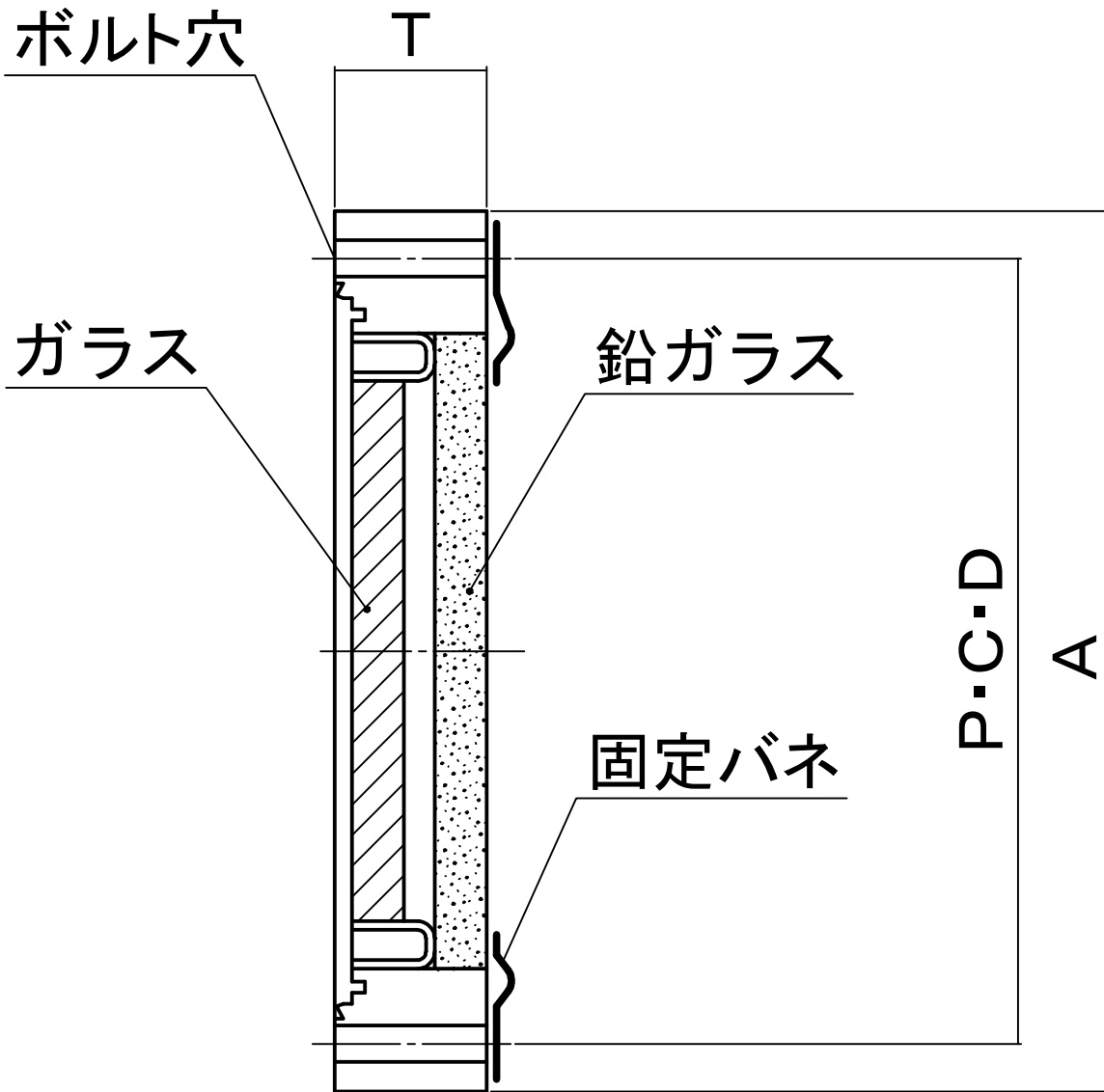
CF 鉛ガラス盤付ガラスビューポート
